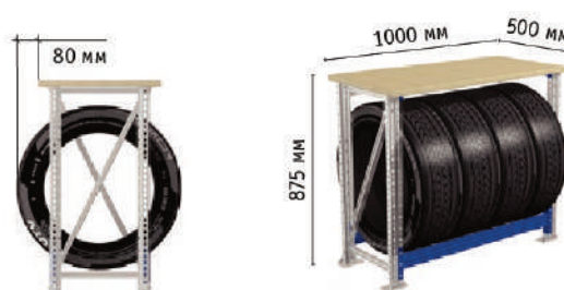
Верстак для хранения автомобильных шин R15 195/65, R16 205/55
